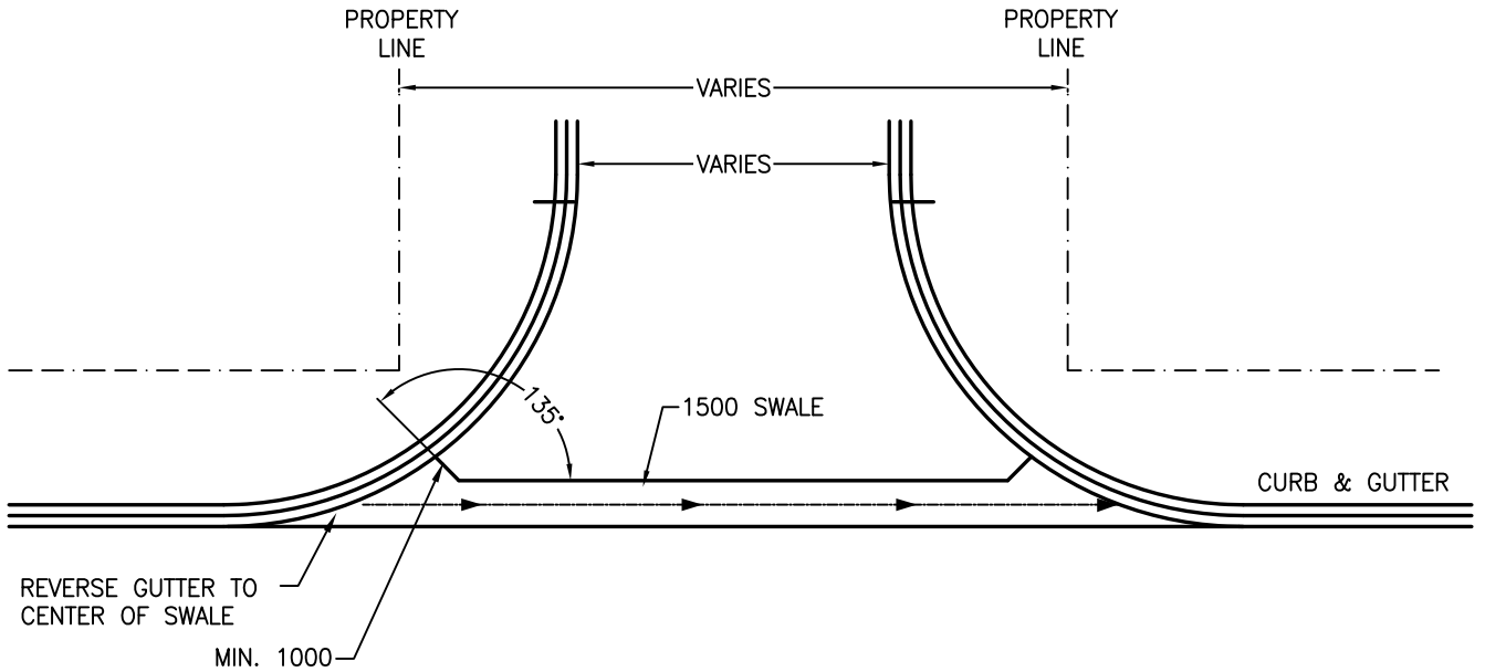
PLAN N.T.S
