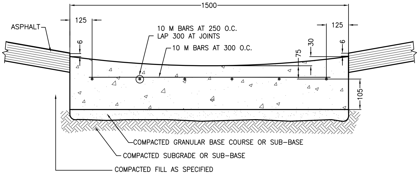
SECTION N.T.S
