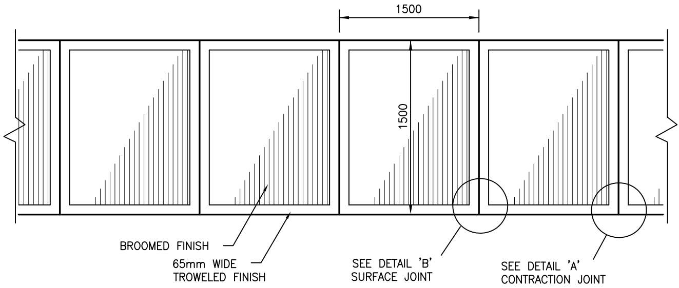
PLAN N.T.S
