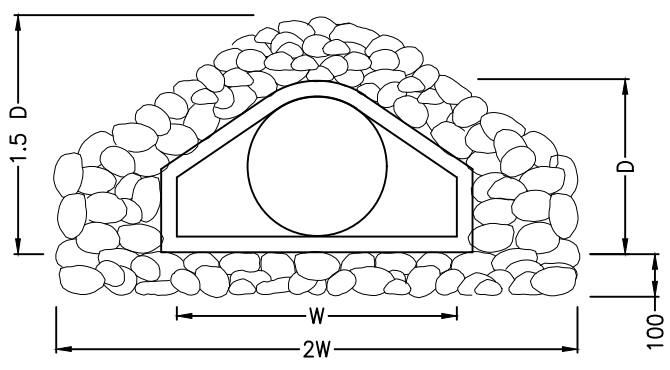
END VIEW N.T.S.
